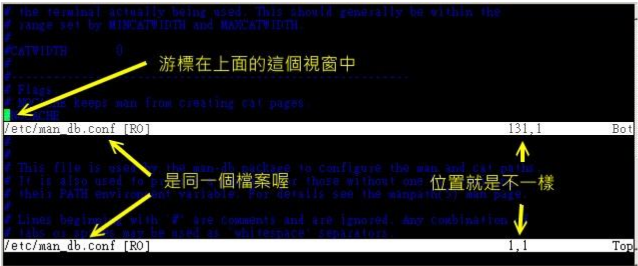
图 9.3.7、vim 的窗口分区示意图
